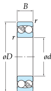
Furo cilíndrico
