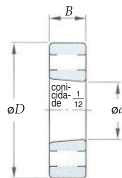
Furo cônico
